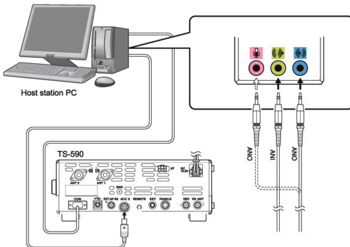
図:4.2.2 音声ケーブルの接続
