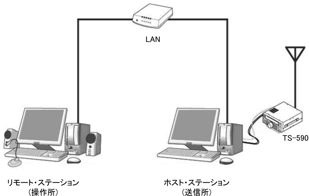
図:3.1.1 家庭内 LAN の構成例
